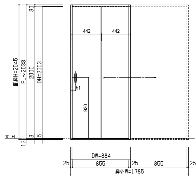
姿図
